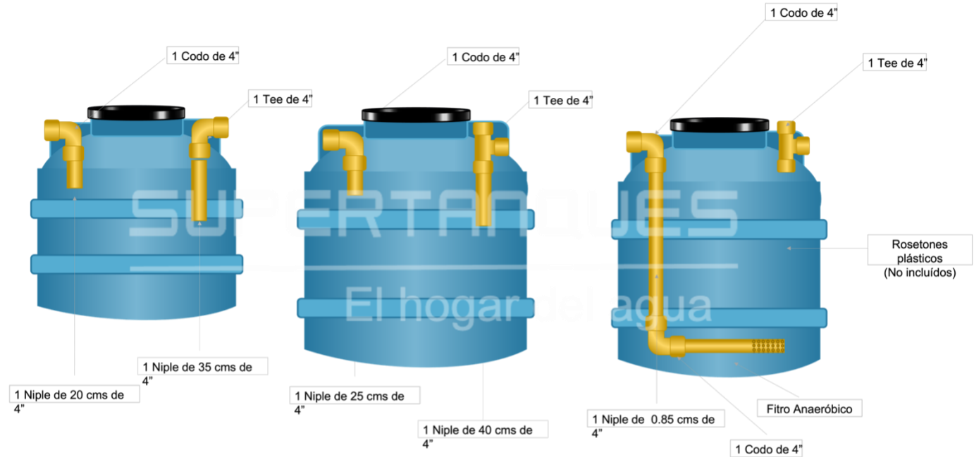
Trampa de Grasa 300L
